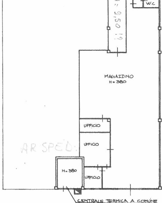
PIANTA DEL PIANO SEMINTERRATO
